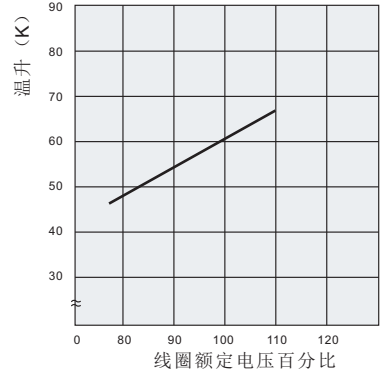
线圈温升
